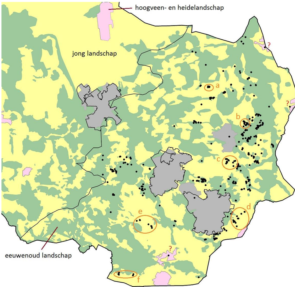
Figuur 3. De verspreiding van Ruige veldbies (opgaven van km hok presentie weggelaten) in Twente geprojecteerd op kaart met onderscheid van jong en eeuwenoud landschap. ? = twijfelachtige opgave, a t/m f = vindplaatsen in jong landschap, a = Asbroek (Achter de Voort), b = Egheria, c = Lonnekerberg, d = Zuid-Eschmarke, e = Asbroek (Twickel), f = Lankheet
