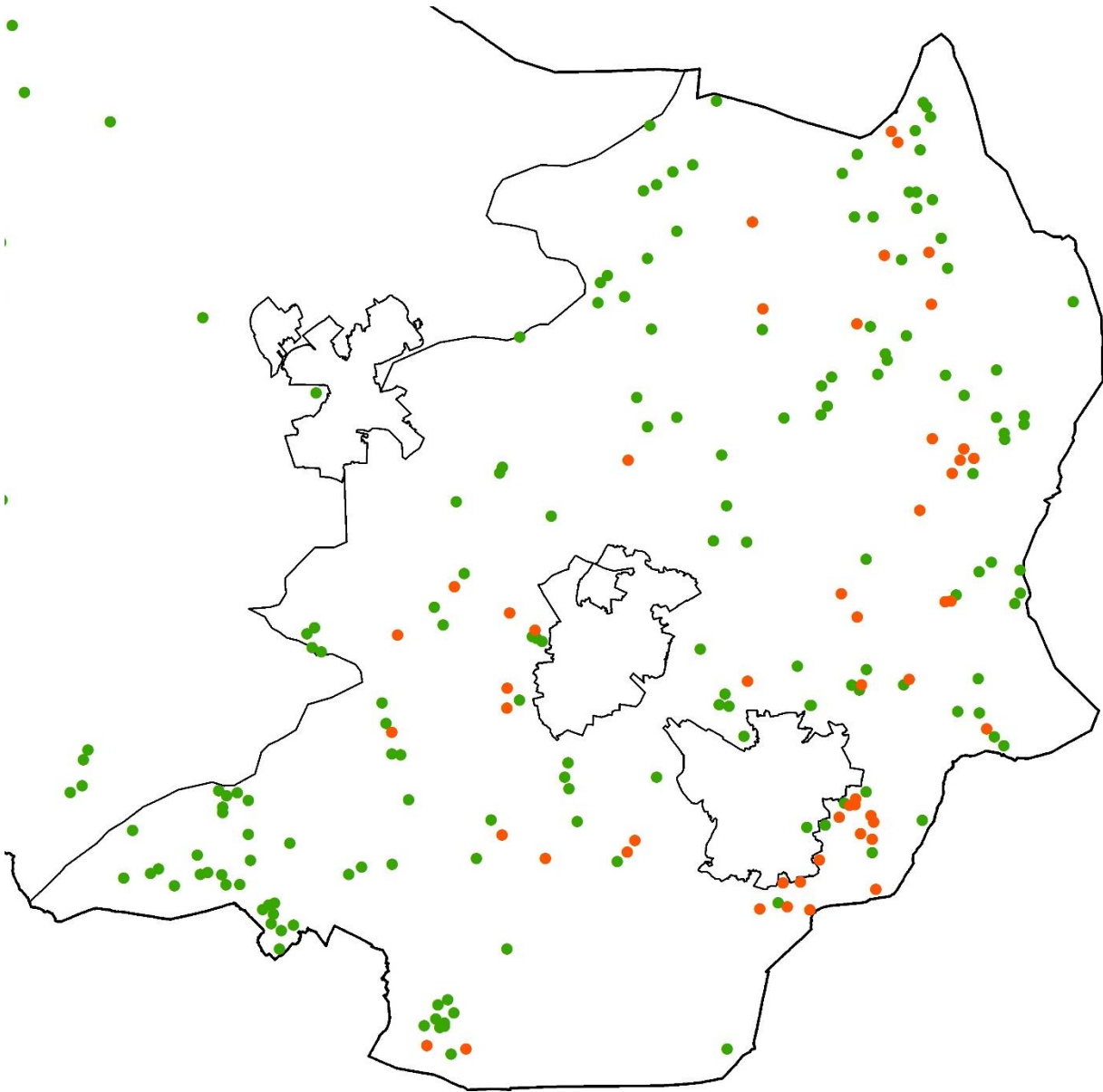
Figuur 2. De verspreiding van eeuwenoude bossen zonder (•) en eeuwenoude bossen met Ruige veldbies (•) in Subcentro-europese floragebied van Twente.
